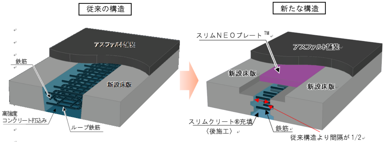
参考図-3 新たなプレキャスト PC 床版の接合構造(大林組提供)
