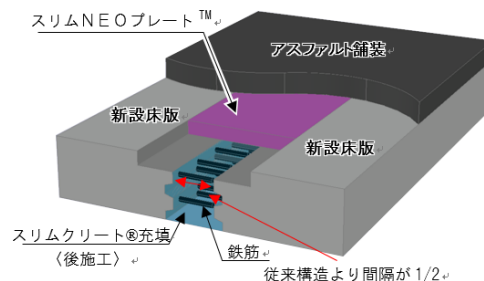
図5 新たなプレキャストPC床版の接合構造(大林組提供)
