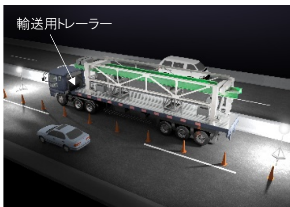
移動式床版架設機の運搬
