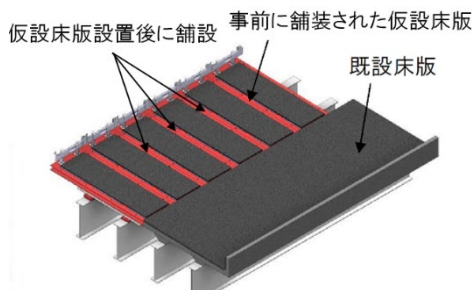
図4 床版取替施工用の仮設床版
