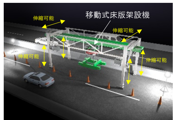
移動式床版架設機の設置
