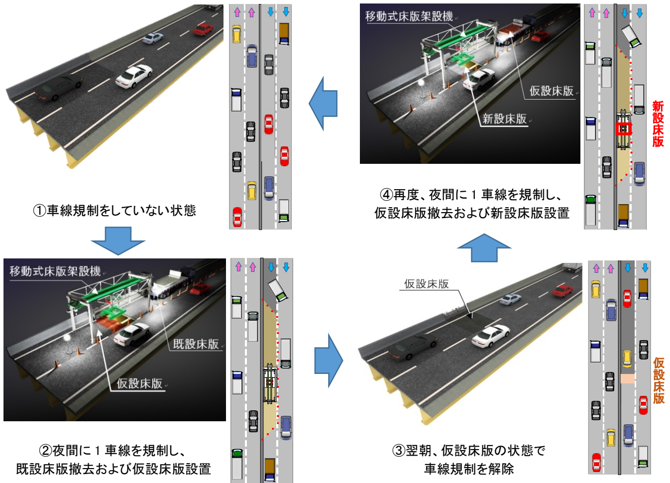
図3 新たな工法による車線規制と施工ステップ(大林組提供)
