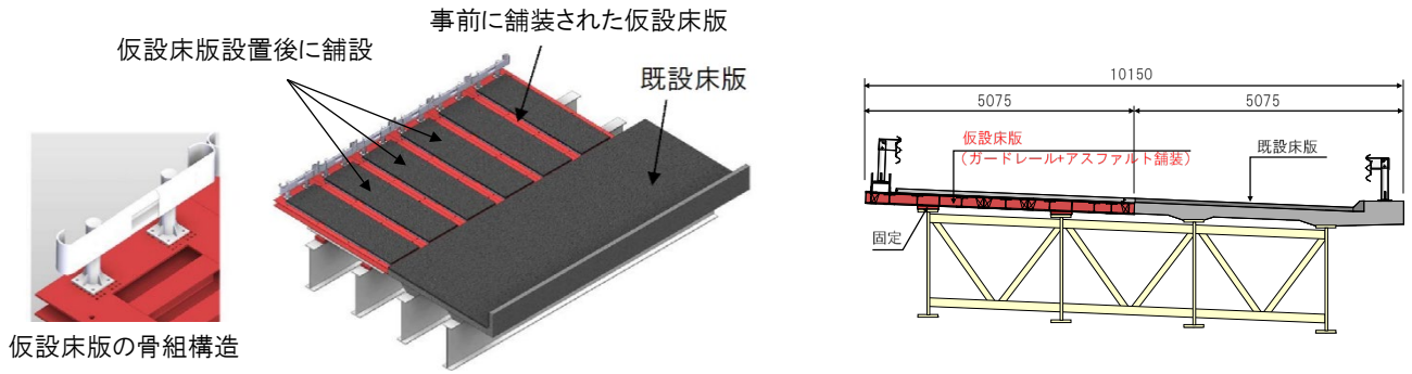
参考図-2 床版取替用の仮設床版の構造
